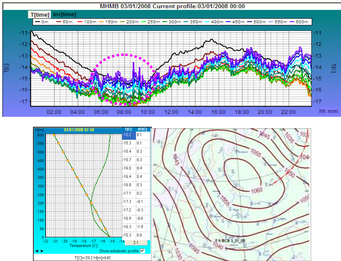
Fig. 27. Turbulence inversion (pink contour).
